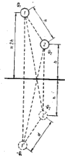
Рис. 13. Схема расположения проводов линии электропередачи
