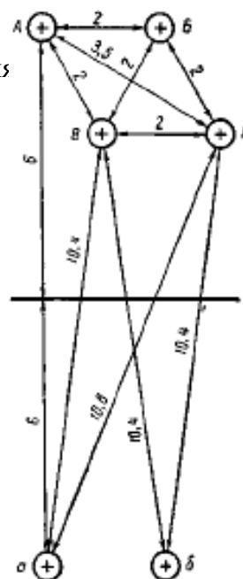
Рис. 14. Схема расположения проводов
