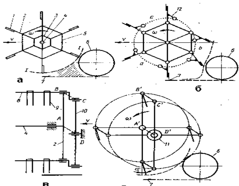
Схемы мотовил:
